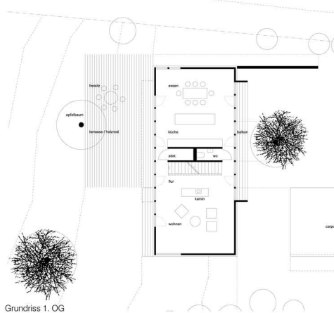
Grundriss 1. OG
