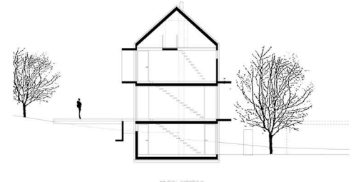
Querschnitt
